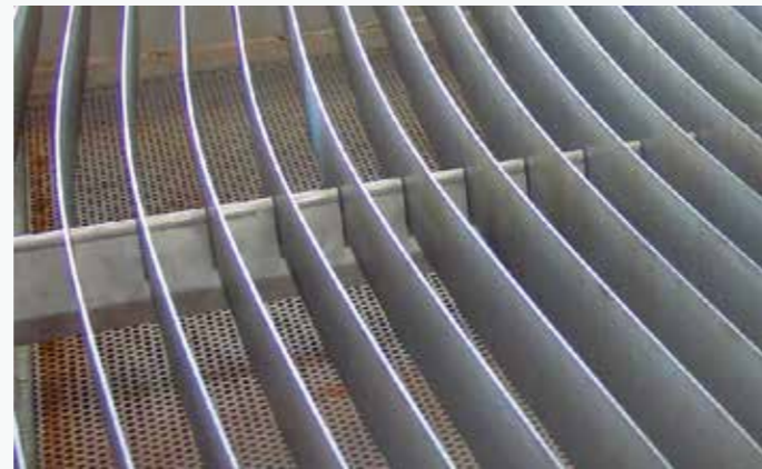
Superficie antirreberveración con platos de chapa dispuestos a 35 o 70 mm (opcional)
