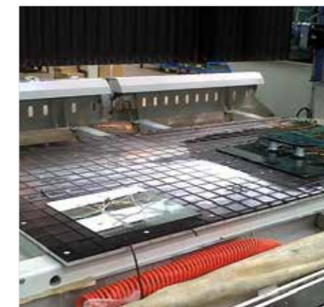
Полностью обрешиненный рабочий стол с вакуумной системой закрепления заготовок
